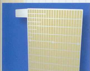
Detail (silná deska s pastou podobnou jako pro užití v trakčních bateriích)
